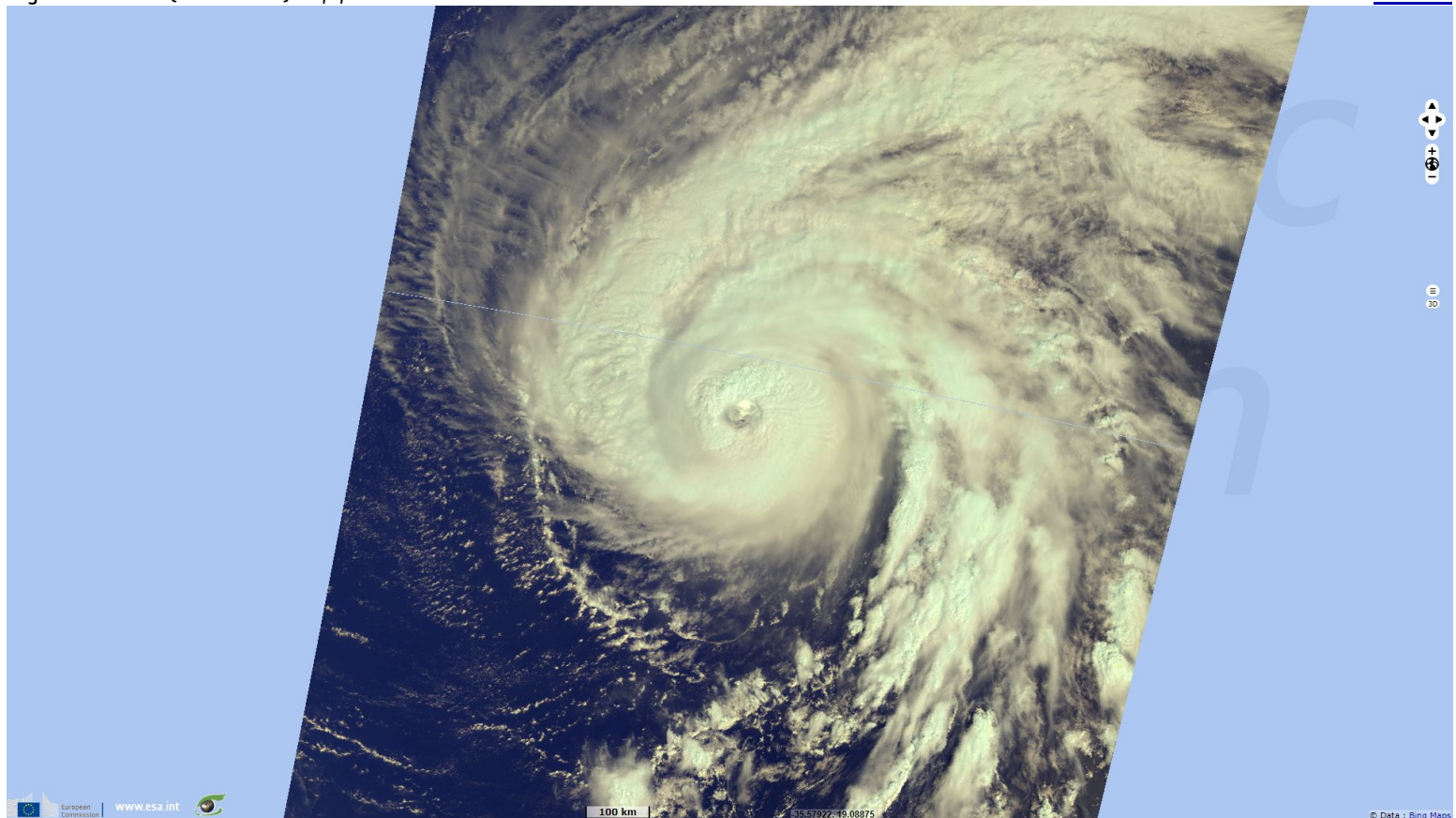
Fig. 4 - S3 OLCI (27.09.2019) 21,9,1.
